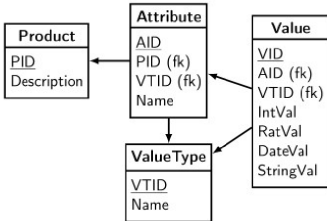
ValueType
